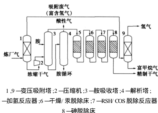
图 1 吸附精馏法工艺流程
